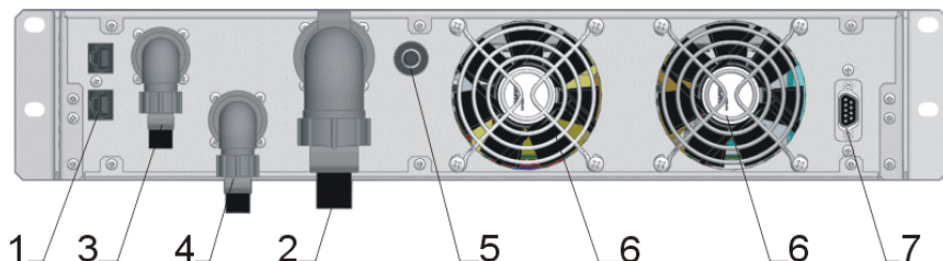
Рис. 2 Задняя панель блока ИБП:
