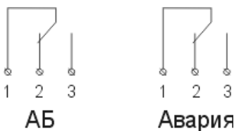
Рис. 5 Сухие контакты ИБП
